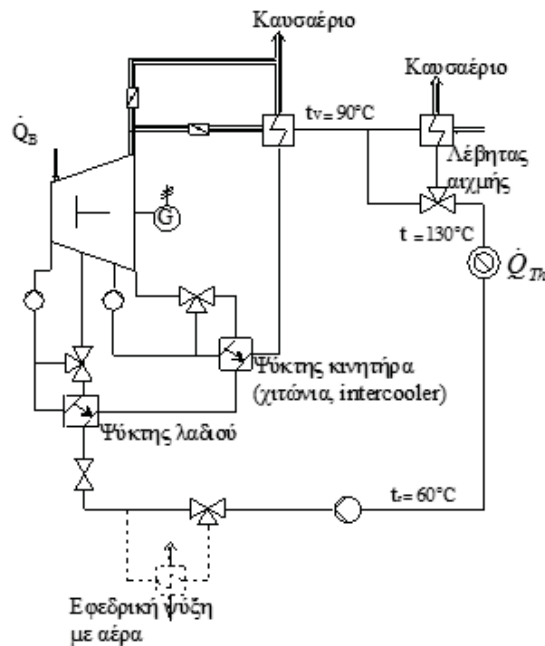
Σχήμα 5 Σύστημα συμπαγωγής με παλινδρομική μηχανή [24]
