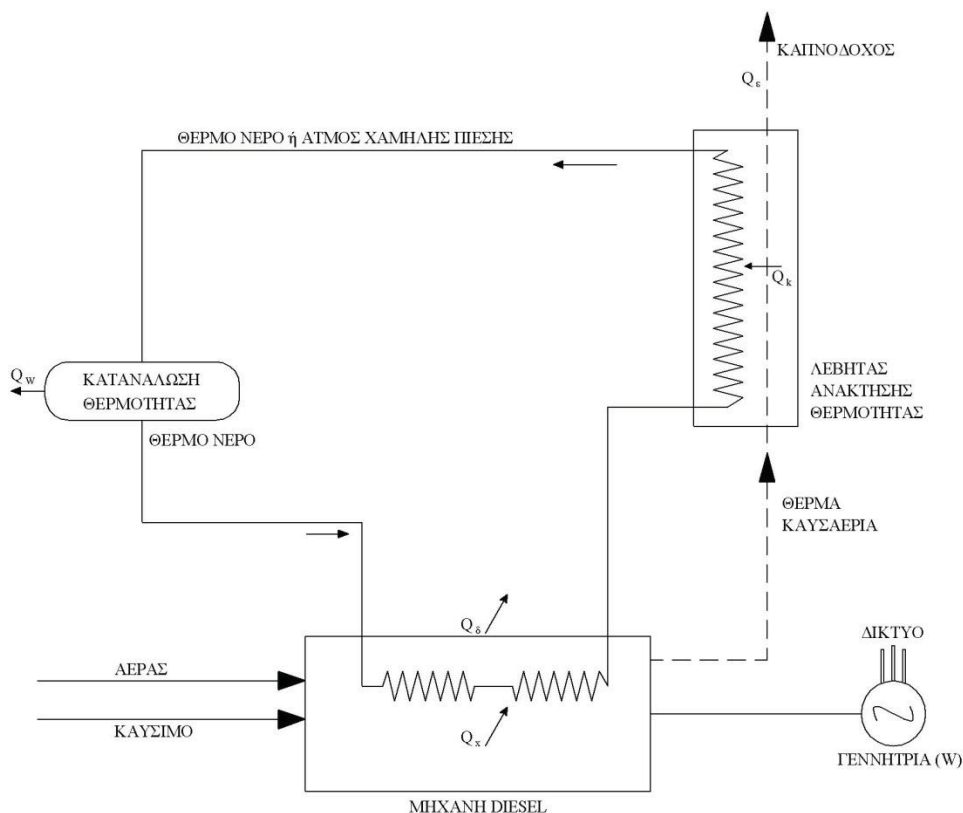
Σχήμα 7 Σχηματικό διάγραμμα συστήματος ΣΗΘ με μηχανή Diesel, εναλλάκτη λαδιού και ψυκτικού νερού χιτωνίων και λέβητα ανάκτησης θερμότητας καυσαερίων, για παροχή ΖΝΧ ή ατμού χαμηλής πίεσης.
